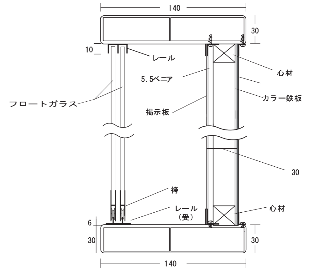
断面図
